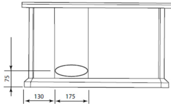
Sicht von hinten rear view
