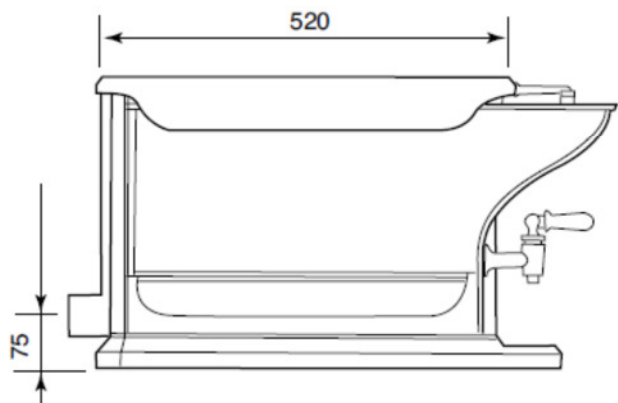
Seltenansicht mit Wasserschiff side view with water tank
