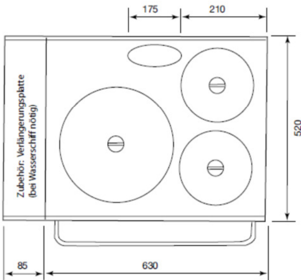
Sicht von oben top view
